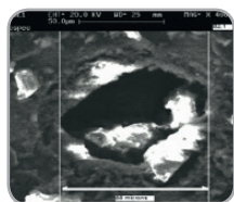
Einspritzöffnung ohne DK Premium nach Langzeittest
