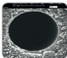
Einspritzöffnung mit DK Premium nach Langzeittest
